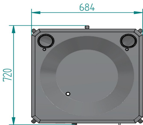
VISTA PLANTA
